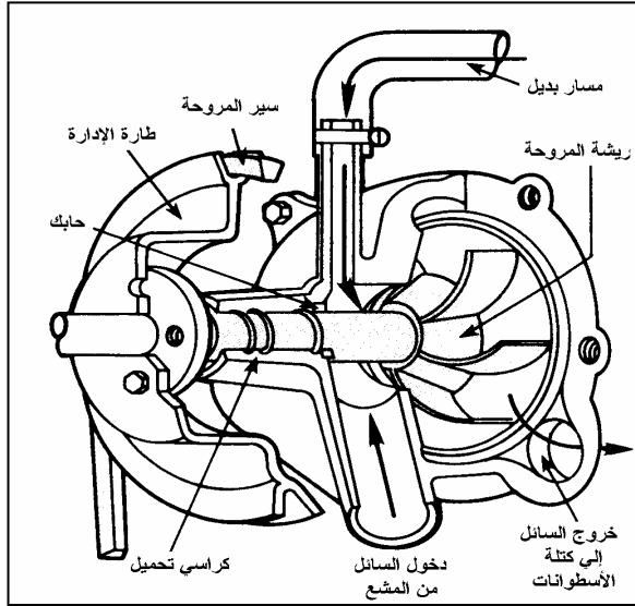
شكل ٣ - ٩ أجزاء مضخة المياه
