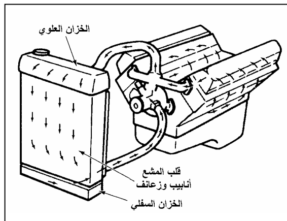
شكل ٣ - ٢ نظام التبريد بالماء
