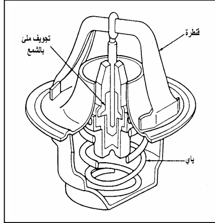
شكل ٣ - ١٠ قطاع
