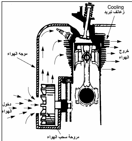
شكل ٢ - ٧ نظام تبريد الهواء
