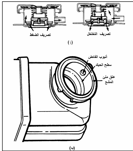
شكل ٣ - ٧- غطاء وعنق ملئ المشع
