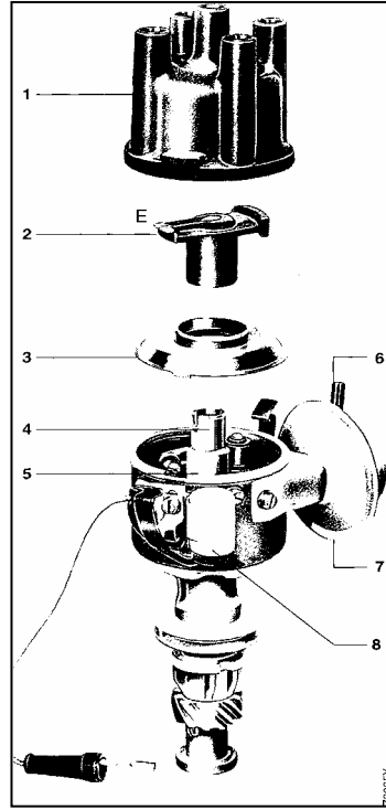
شكل ٥ - ٤ أجزاء موزع الشرر
