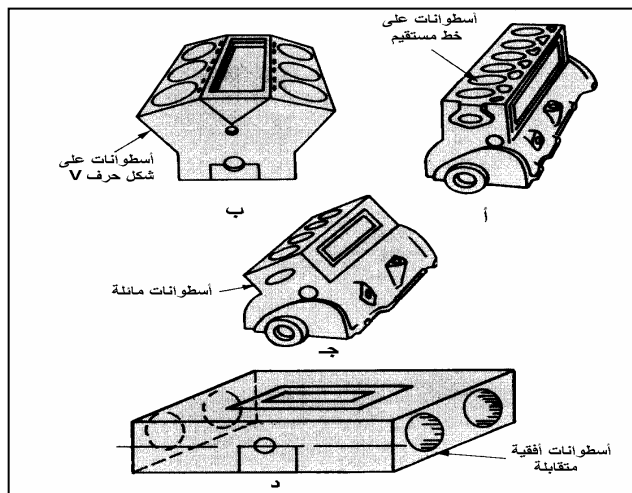
شكل ٢ - ٣ الأشكال المختلفة لترتيب الأسطوانات بالمحرك
