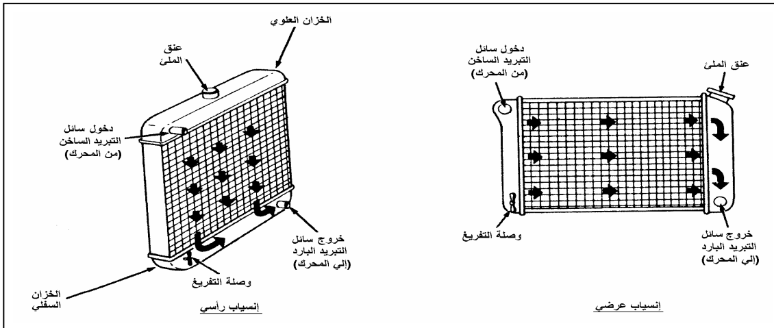
شكل ٦- ٣ التصميمات المختلفة للمشع (أ - انسياب عرضى، ب - انسياب رأسى)
