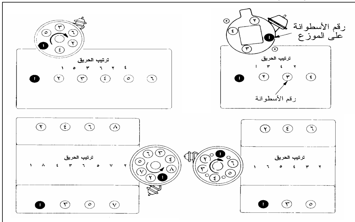
شكل ٢ - ٤ الأشكال الشائعة لترقيم الاسطوانات وترتيب الحريق (الاشعال)
