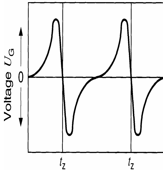
شكل ٥ - ١٧ توليد القوة الدافعة
