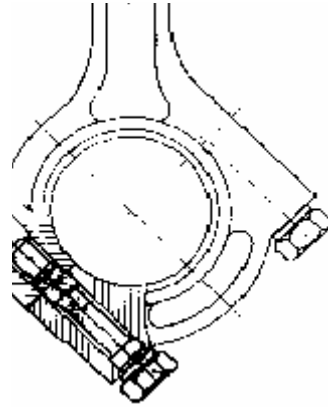
شكل ١ - ١٩ يوضح ذراع التوصيل بنهاية كبرى مائلة
