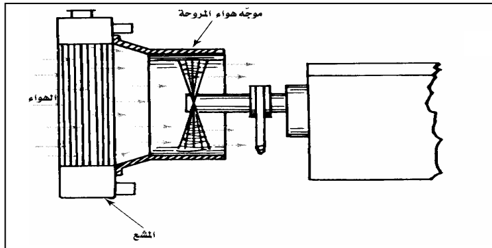
شكل ٣- ١٧ موجّه هواء المروحة
