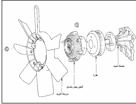
شكل ٣- ١٥ أجزاء المروحة التي بها قابض
