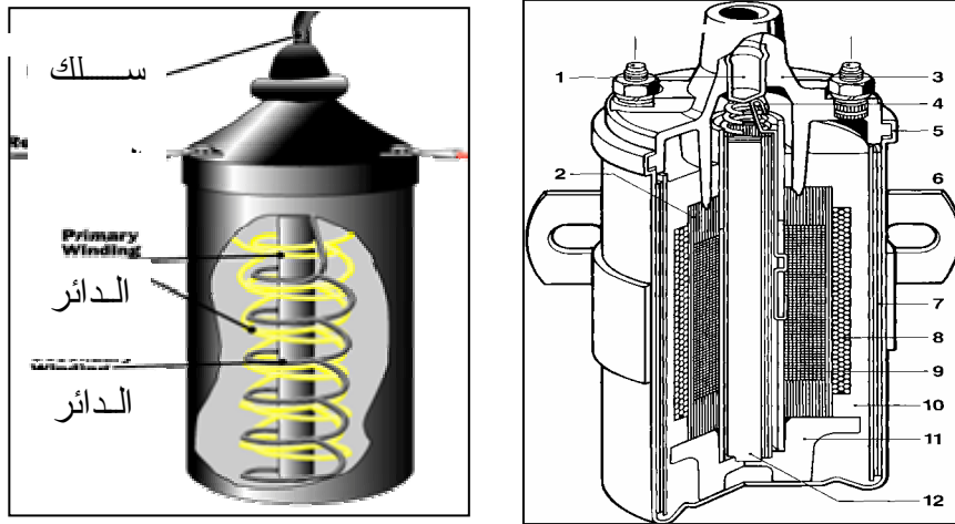
شكل ٥ - ٣ مكونات ملف
