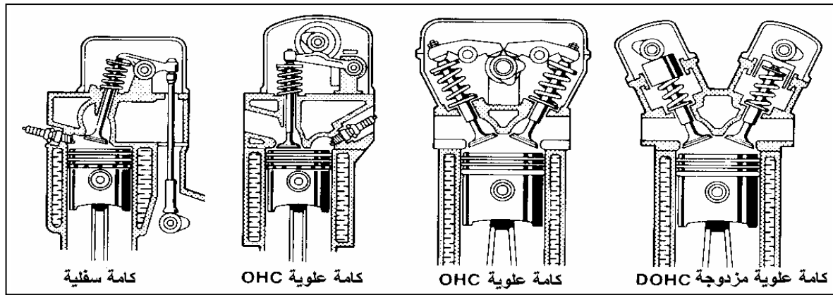
شكل ٢ - ١٠ وضع وتركيبية عمود الكامات بالمحرك
