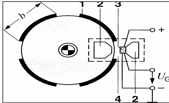
شكل ٥ - ١٩ أجزاء نظام مولد هول.
