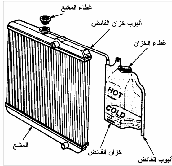
شكل ٣ - ٨ النظام المغلق مع خزان الفائض
