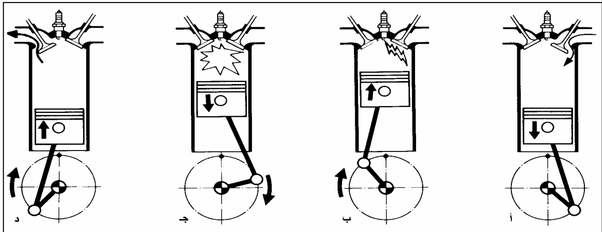
شكا، ٢- ١- الدورة الرباعية
