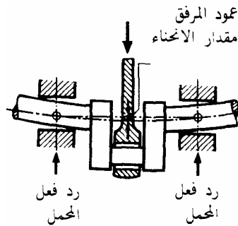
شكل ٢٢ - ١ يوضح إجهاد الحني على عمود المرفق
