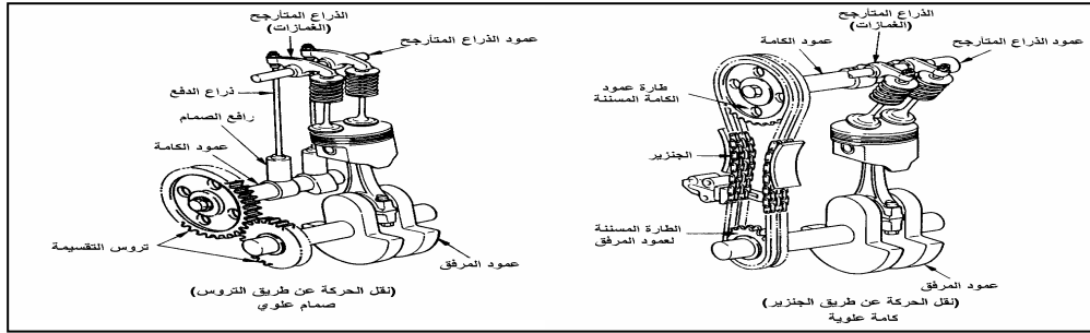
شكل ٢ - ٩ نقل الحركة عن طريق الجنزير للكامات العلوية ونقل الحركة عن طريق التروس
