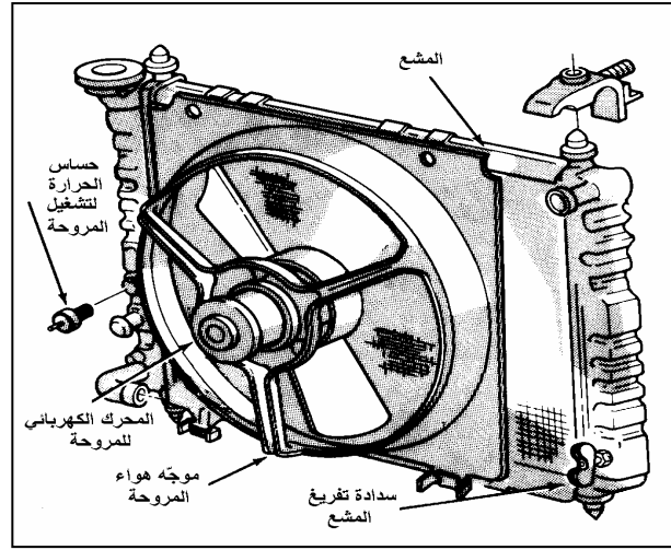
شكل ٣- ١٦ إدارة المروحة عن طريق المحرك الكهربائي،
