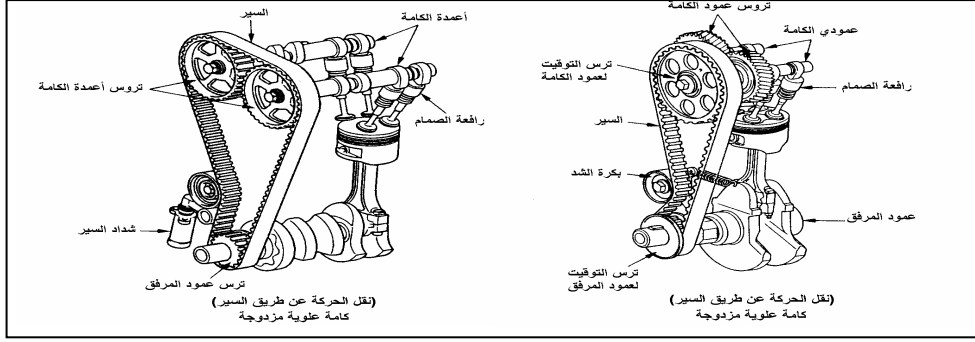
شكل ٢ - ٨ نقل الحركة لعمود الكامات عن طريق
