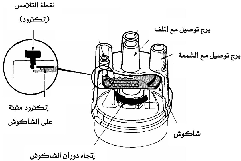
شكل ٥ - ٥ غطاء الموزع والشاكوش
