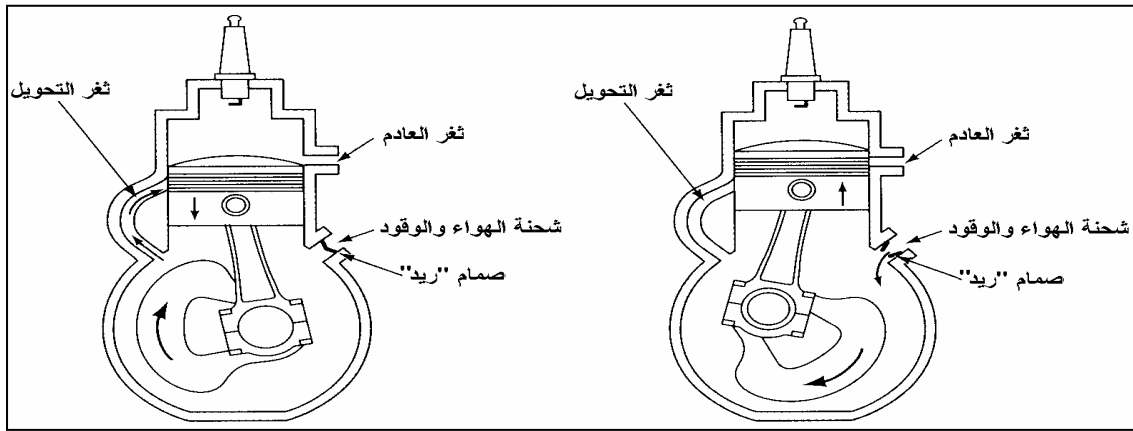
شكل ٢ - ٢ الدورة الثنائية
