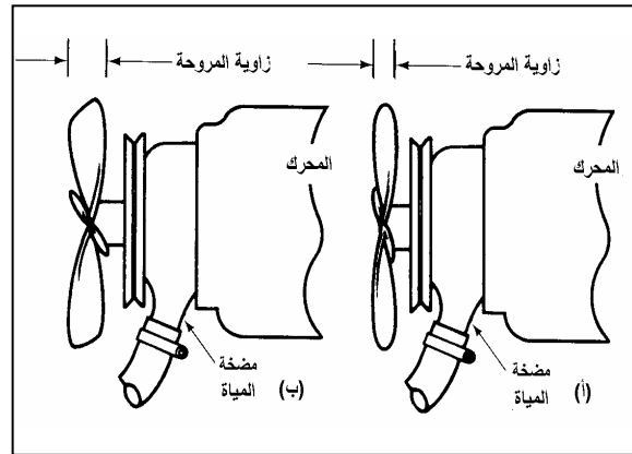
شكل ٣- ١٤ سرعة دوران المروحة أ) سريعة ، ب) بطيئة
