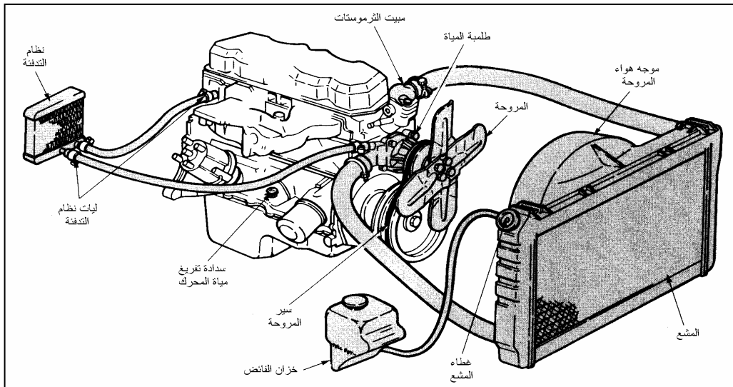
شكل ٣ - ٣ أجزاء نظام التبريد
