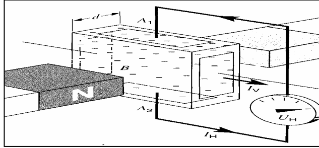
شكل ٥ - ١٨ مبدأ مولد هول.
