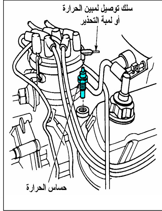
شكل ٣- ١٩ مكان توصيل حساس الحرارة
