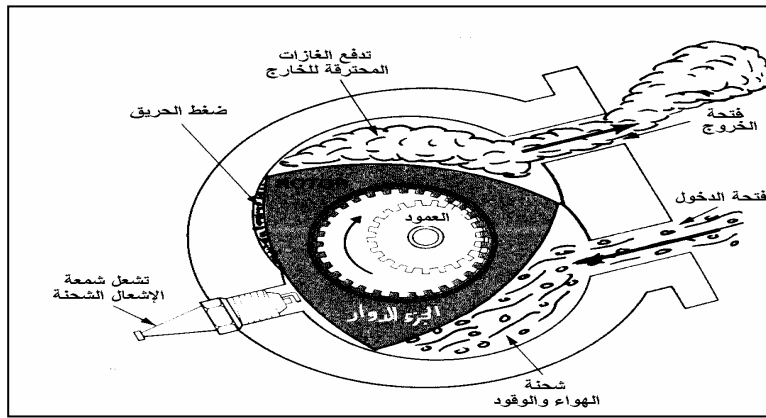
شكل ٢ - ١٥ شكل وأجزاء المحرك الدوار
