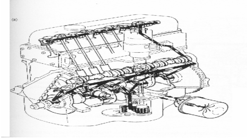
شكل (٤ - ١) دورة الزيت في المحرك
