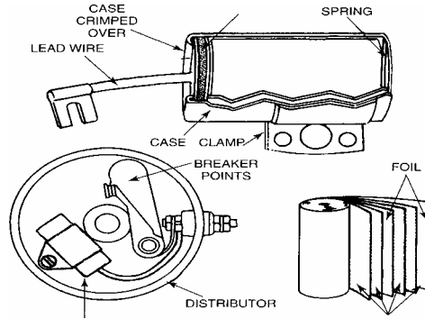
شكل ٥ - ٩ أجزاء المكثف.
