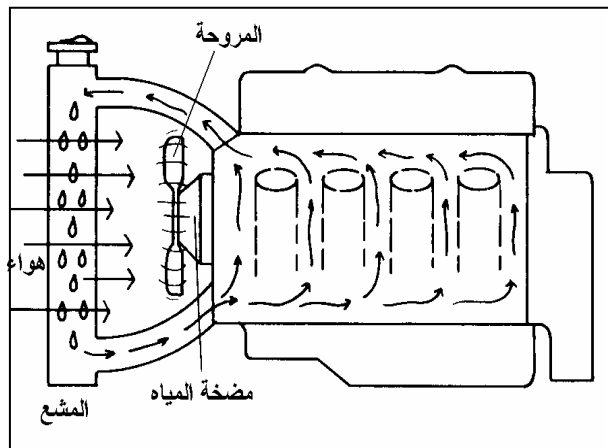
شكل ٢ - ٦ نظام تبريد المياه
