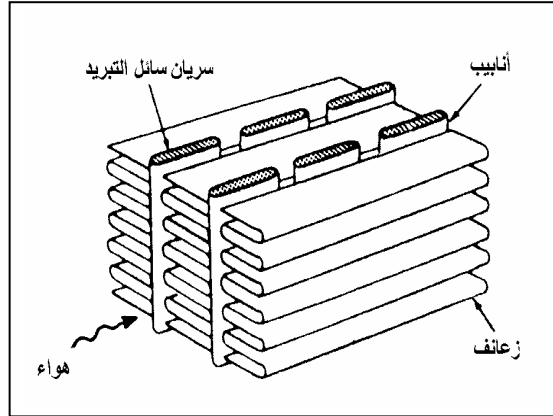
شكل ٣- ٥- مقطع بالمشع
