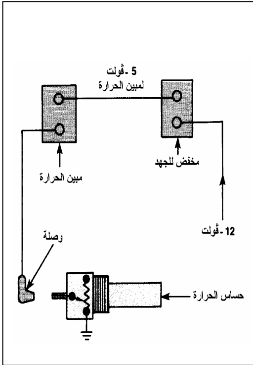
شكل ٣- ٢٠ الدائرة الكهربائية لمبين الحرارة
