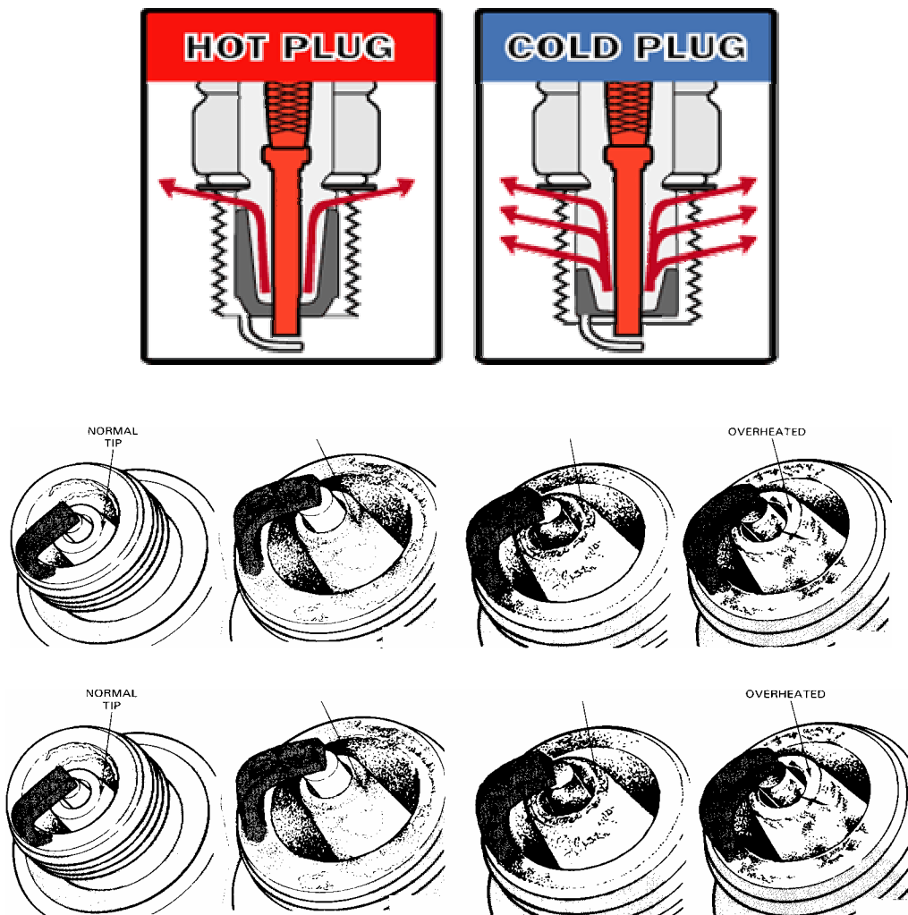
شكل ٥ - ١٠ شمعات الساخنة و الباردة
