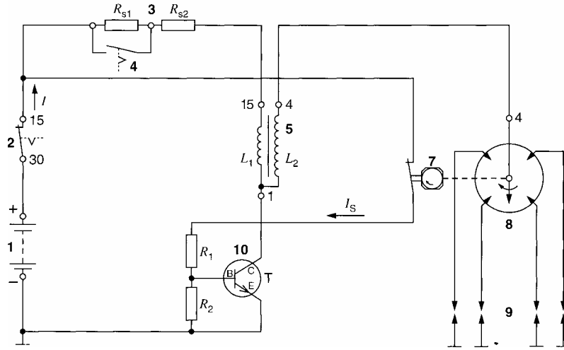
شكل ٥ - ١٣ دائرة التوصيل لمجموعة الإشعال الترنزستوري. البطارية.
