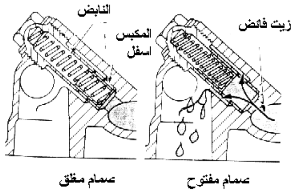
شكل (٤ - ٤) صمام ضغط الزيت مغلق ومغلق
