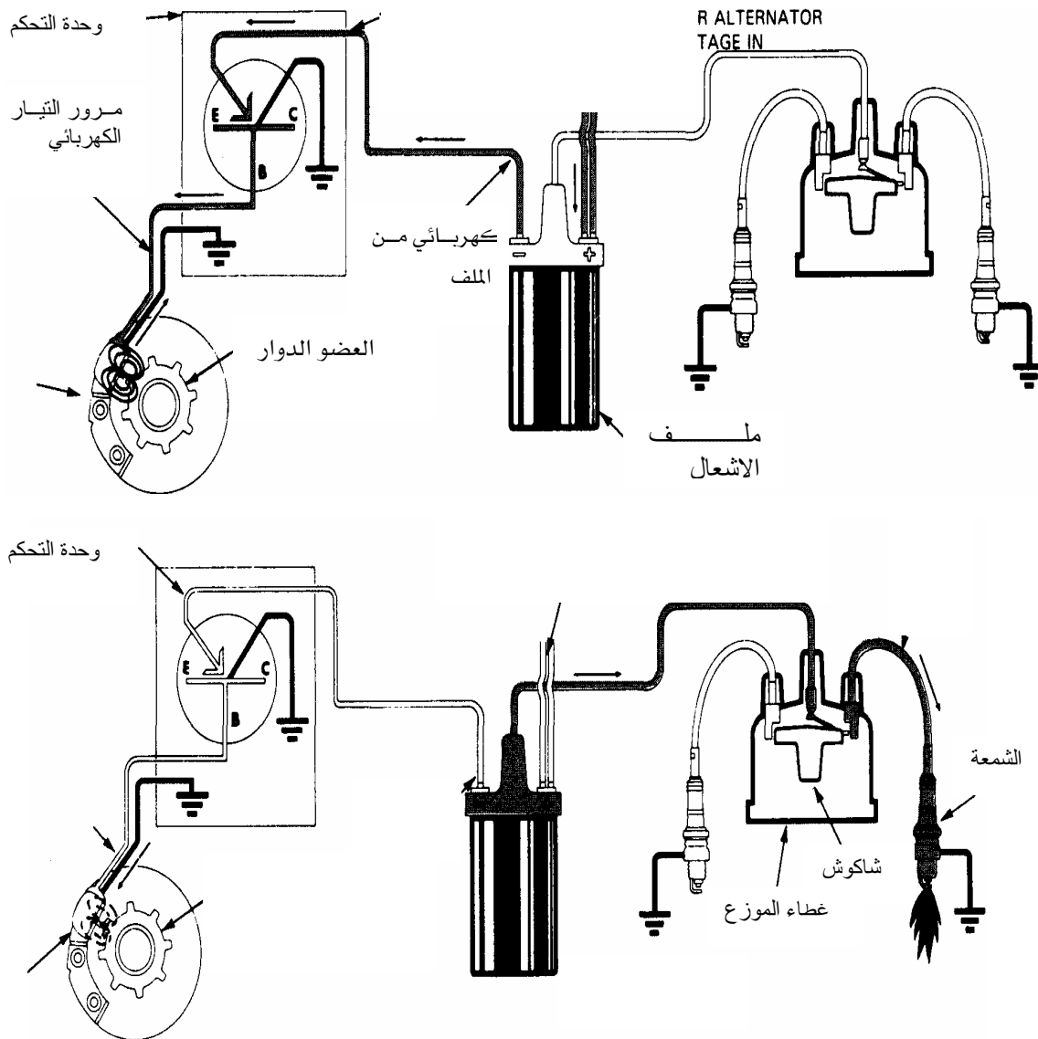
شكل ٥ - ١٥ نظام الإشعال الإلكتروني بمولد النبضة الحثي.
